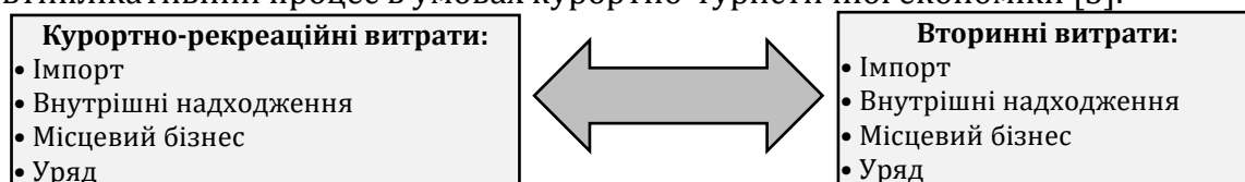
Рис. 3. Мультиплікативний процес
