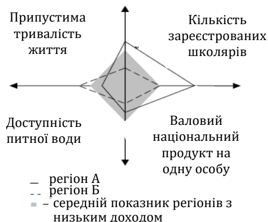
Рис. 2. Порівняння двох регіонів за методом «ромбів»
